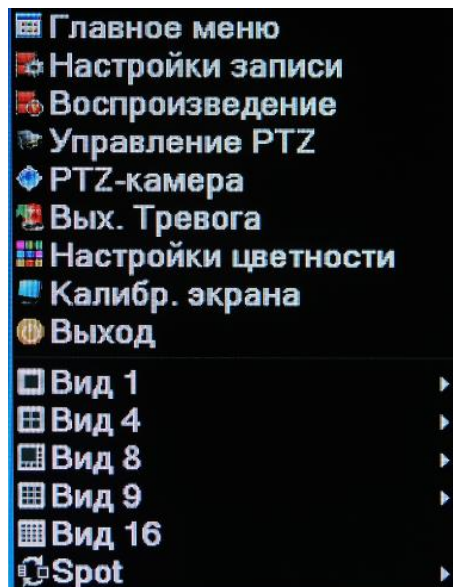
Рис. 3.1. Всплывающее меню
