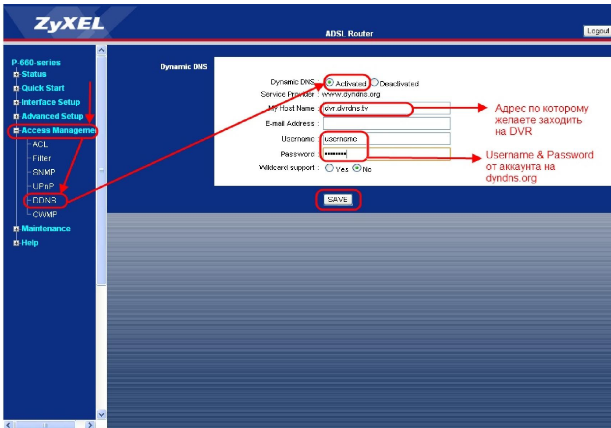
Рис. 6.9. Настройки маршрутизатора
