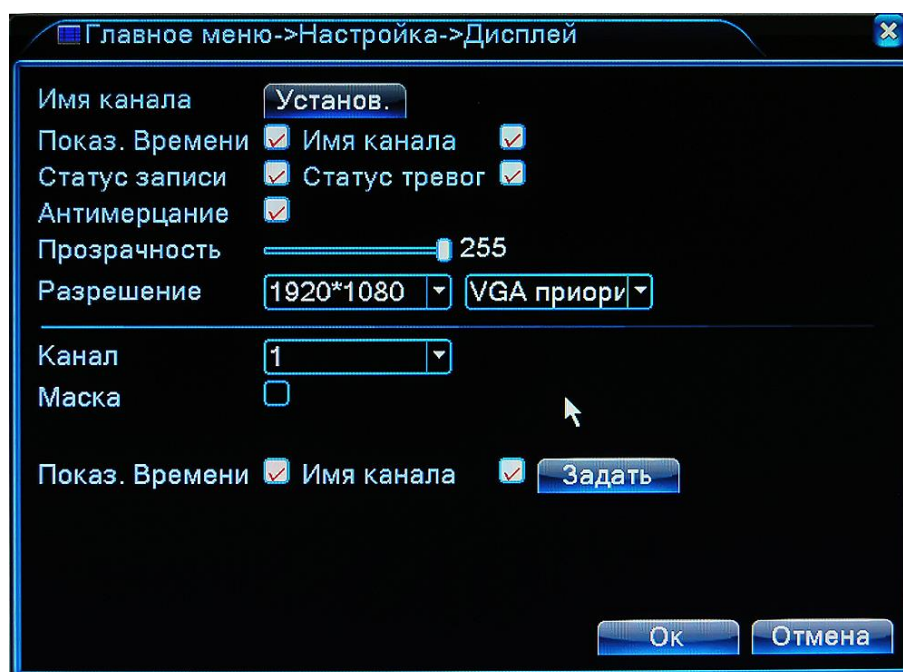
Рис. 4.3.5.1. Настройка. Дисплей
