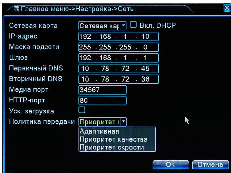
Рис. 4.3.3.1. Настройка. Сеть
