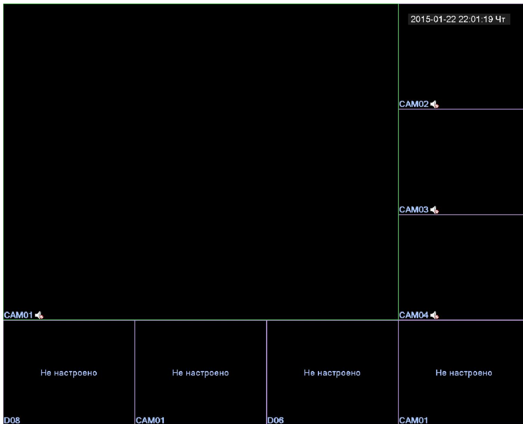
Рис.2.1.2. Режим «Вид 8»
