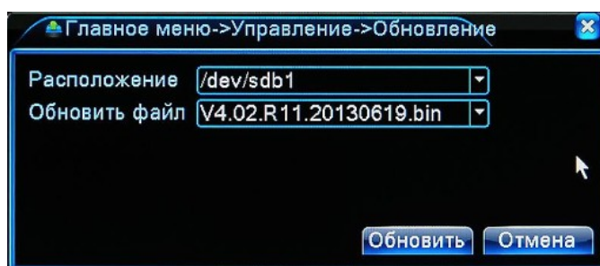
Рис. 4.4.3. Управление. Обновление
