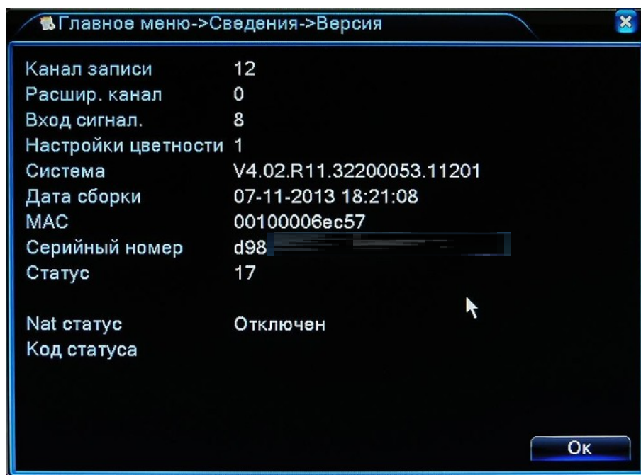
Рис. 4.5.4. Управление. Версия
