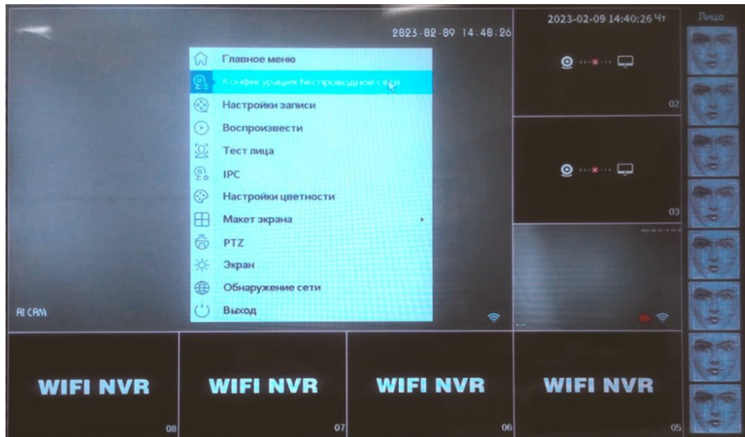
Рис. 3.1. Всплывающее меню
