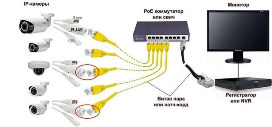
СТАНДАРТНАЯ СХЕМА ПОДКЛЮЧЕНИЯ IP-КАМЕР К РЕГИСТРАТОРУ
