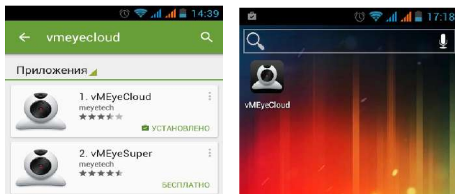
Рис. 7.1.1. Приложение vMEyeCloud
